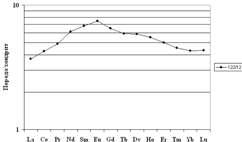
Рис. 3. График распределения РЗЭ для породы меланократового прослоя (обр. 122/12) интрамагматической дайки. Нормирование на хондрит C1 [Sun & McDonough, 1989].
