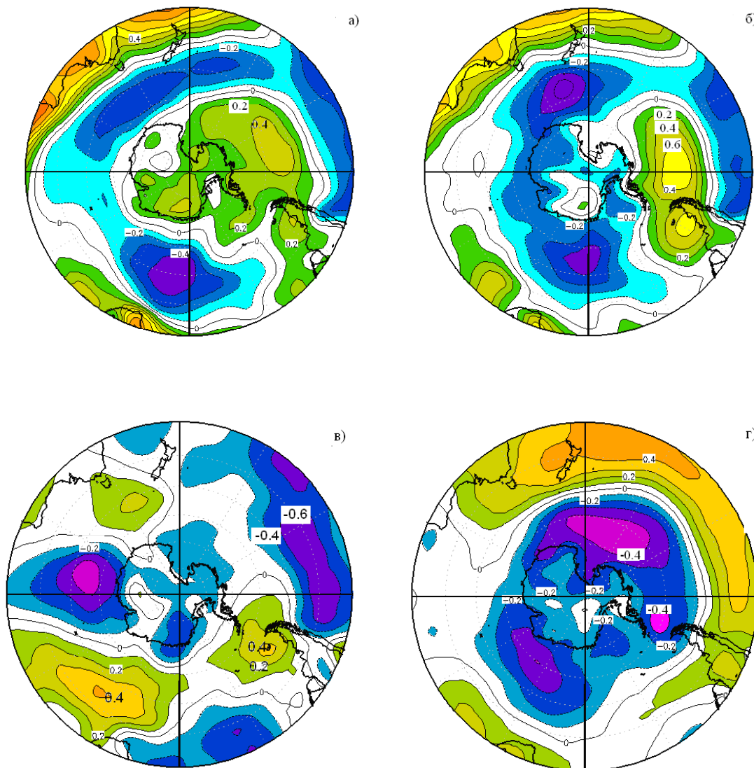
Рис. 3. Пространственная корреляция индекса Эль-Ниньо 1-2 с полем атмосферного давления, сетка 2.5°, 1971-2010, реанализ NCEP-NCAR. а)- синхронная корреляция, декабрь-февраль, б), в), г) — асинхронная, с временным смещением поля давления на 3, 6 и на 9 мес., соответственно
