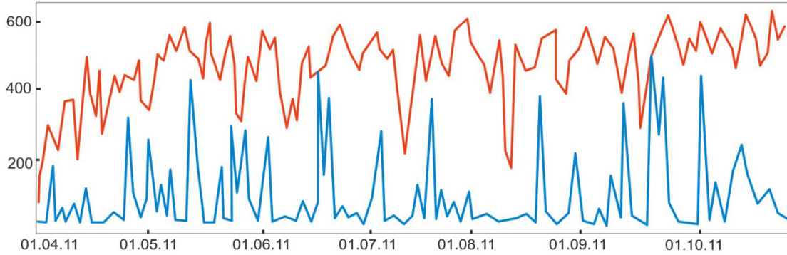
Рис. 4. Варіації значень показників F-статистики для ряду систолічного тиску(згори) і ряду рівня інфразвуку (внизу).
