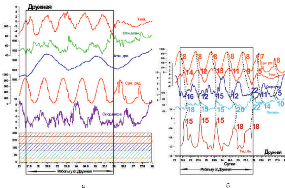
Рис. 6. Временной ход: а - температуры воздуха, относительной влажности, атмосферного давления, суммарной радиации, скорости и направления ветра; б - тех же параметров (кроме атмосферного давления и направления ветра) и температуры воды в период многочасовых зондирований у станции Дружная. Цифры на рисунке (б) обозначают время (в часах) наступления максимумов разных параметров.
