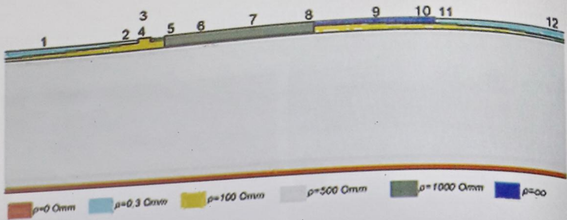
Рис. 6. Реальний розріз робочого профілю моделі
