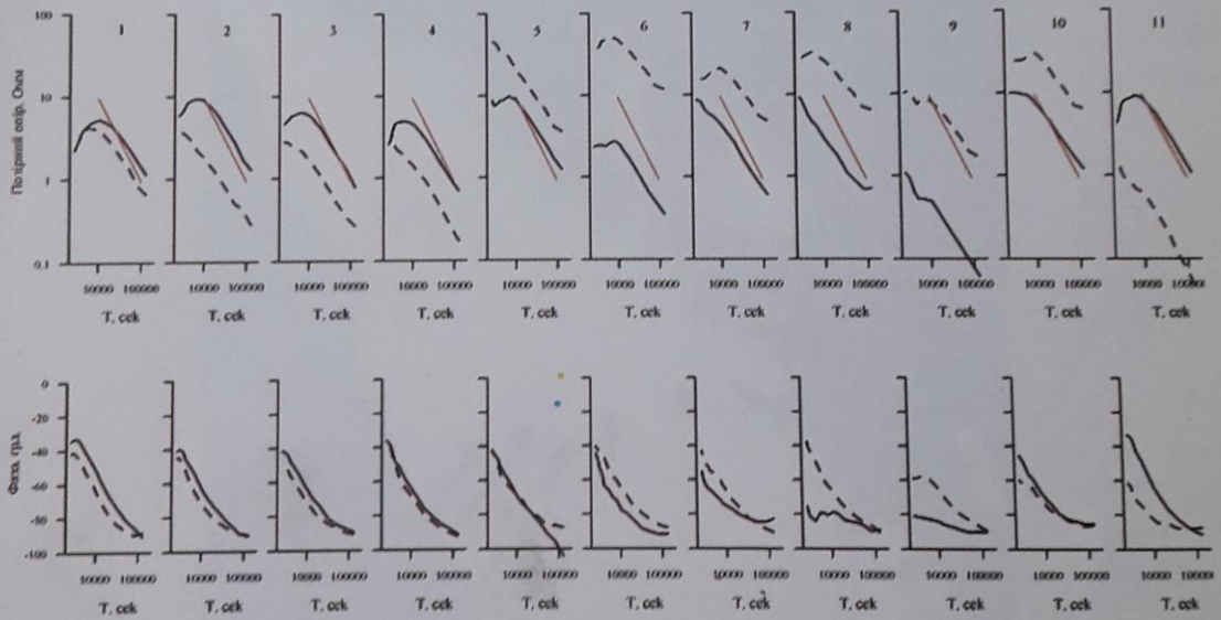
Рис. 3. Амплітудні та фазові криві МТ зондування в пунктах 1-11. Суцільна лінія - R_{xy} , пунктир - R_{yx} , червона - R_n
