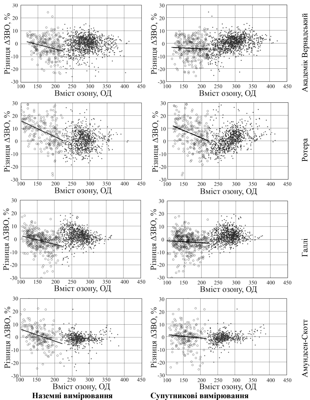
Рис. 3. Залежність відносної різниці \Delta ЗВО від рівня ЗВО, одержаного за наземними (ліворуч) та супутниковими (праворуч) вимірюваннями. Кругками позначено спостереження в період озонної діри, точками – після її розпаду.
