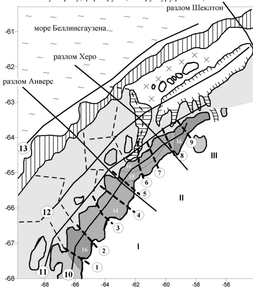
Рис. 1. Структурно-тектоническая схема района Антарктического полуострова (Земля Грейама). Поперечные разломы Антарктического полуострова: 1 – Лаллеманд; 2 – Дарбел; 3 – Барилари; 4 – Бескочае; 5 – Фландрес; 6 – Брабант; 7 – Палмер; 8 – Тринити; 9 – Расселл. Продольные разломные зоны на Антарктическом полуострове и его западном шельфе: 10 – линия свода гор Антарктического полуострова; 11 – внутреннего шельфа; 12 – внешнего шельфа; 13 – основания материкового склона; I, II, III – сектора Антарктического полуострова и континентальной окраины, ограниченные разломами Анверс, Херо и Шеклтон.
