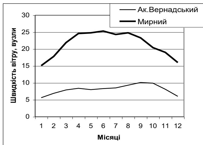
Рис. 4. Річний хід швидкості вітру.
